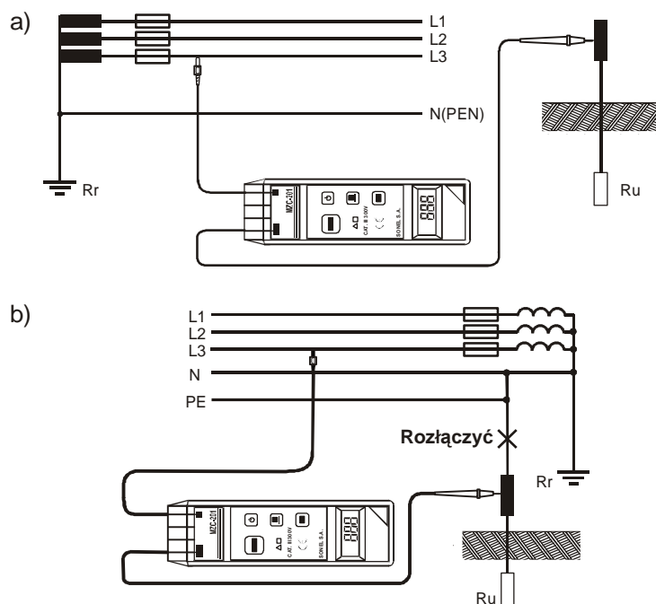
Rys.10. Sposób podłączenia miernika z rodziny MZC-200 przy pomiarach rezystancji uziemień: a) dla sieci TN-C, TN-S i TT, b) dla sieci TN-C-S
